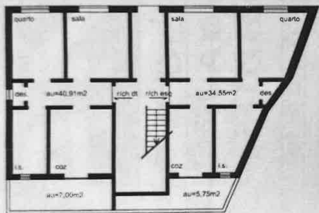
PLANTA R/CH
