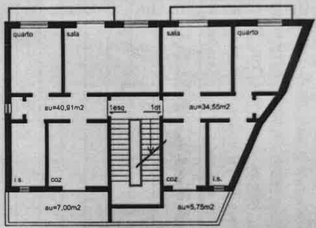
PLANTA PISO 1
